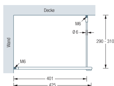
G400HD Seitenansicht:
