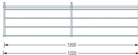
G1-1200 Draufsicht:
