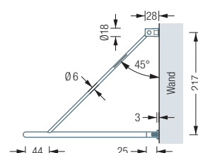
GU1-1600 Seitenansicht:
