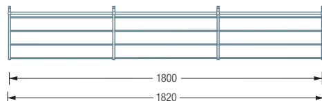
G1-1800 Draufsicht:
