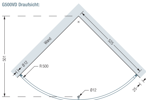
G500VD Draufsicht:
