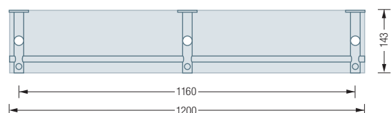
G4-1200 G/H/CDF/CDFD Draufsicht:
