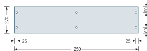
Ablage G3-1200 G / H / CDF / CDFF Draufsicht:
