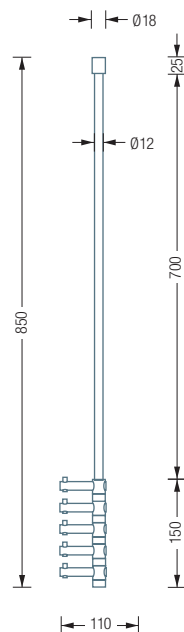
T5 Seitenansicht:
