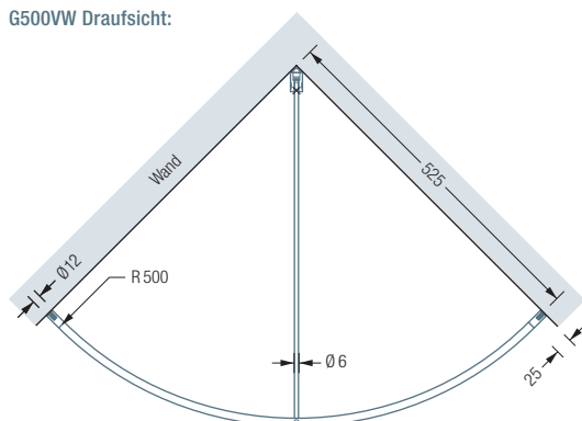
G500VW Draufsicht:
