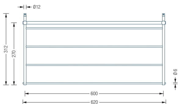
G1-600 / 1200 / 1800 Seitenansicht:
