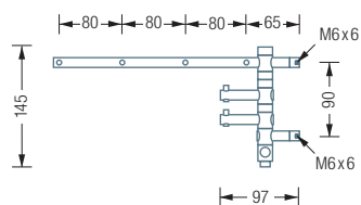
G1-600 / 1200 / 1800 Seitenansicht:
