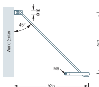
G500VW Seitenansicht:
