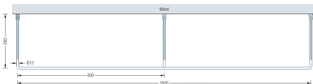
GU1-1600 Draufsicht:
