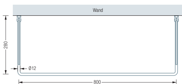
GU1-800 Draufsicht:
