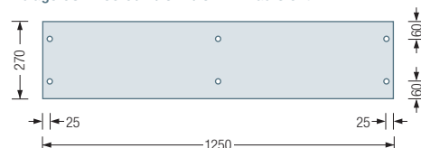
Ablage G8-1200 G/H/CDF/CDFF Draufsicht:
