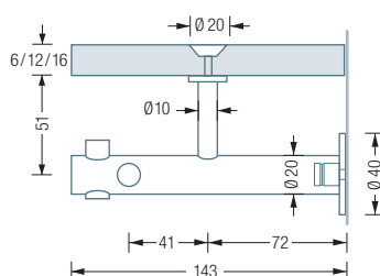
G4-600/1200 G/H/CDF/CDFD Seitenansicht:
