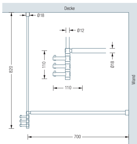
Deckenmontage mit Deckenlager DL12:
