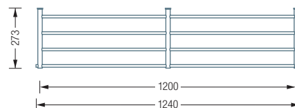
G8-1200 Draufsicht:
