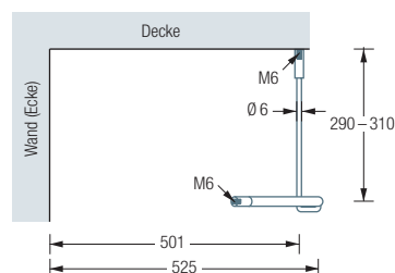
G500VD Seitenansicht:
