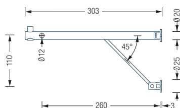
G3-600 / 1200 Seitenansicht:
