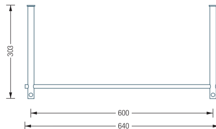
Ablage G3-600 G / H / CDF / CDFF Draufsicht:
