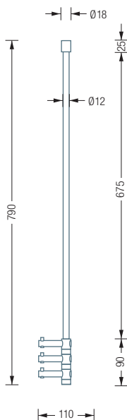
T3 Seitenansicht:
