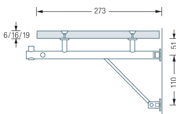
G3-600 / 1200 G / H / CDF / CDFF Seitenansicht:
