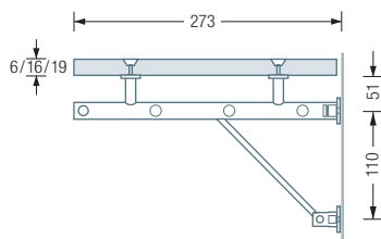
G5-600 / 1200 G / H / CDF / CDFD Seitenansicht:
