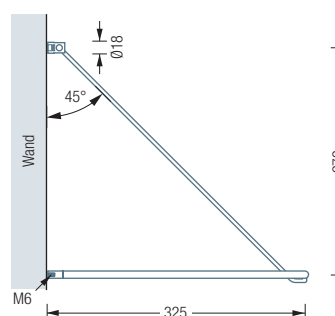
G300HW Seitenansicht:
