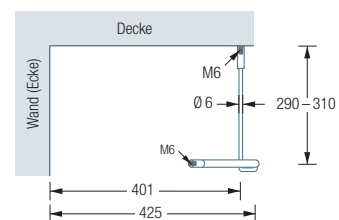
G400VD Seitenansicht:
