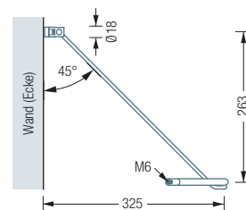
G300VW Seitenansicht:
