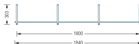
G3-1800 Draufsicht:
