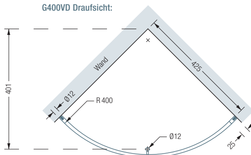
G400VD Draufsicht:
