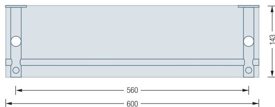
G4-600 G/H/CDF/CDFD Draufsicht:
