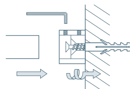
Wandmontage mit Wandlager WL18:
