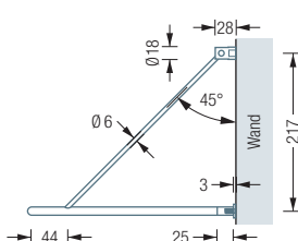
GU1-800 Seitenansicht:
