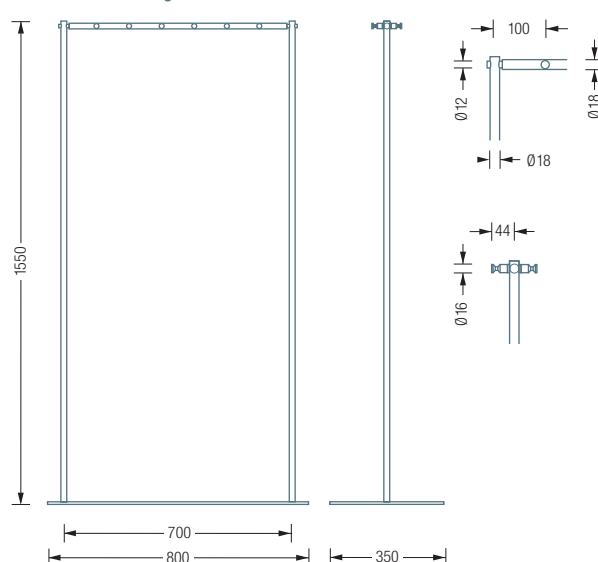
GST3 mit Hakenstange:
