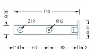
G7-600/-1200/-1800 Seitenansicht:
