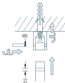
Deckenmontage mit Deckenlager DL12:
