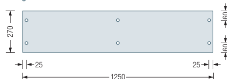
Ablage G5-1200 G / H / CDF / CDFD Draufsicht:
