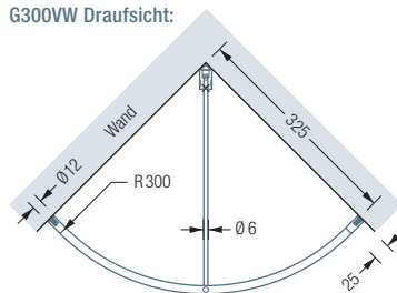
G300VW Draufsicht:
