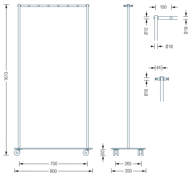
GW2 mit Hakenstange:
