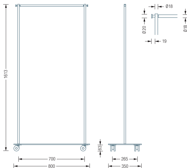
GW1 mit Kleiderstange:
