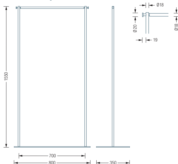
GST2 mit Kleiderstange:
