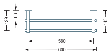
G7-600 Draufsicht:
