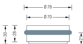
TSB70-30 Seitenansicht:
