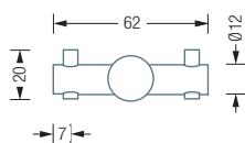
H18-50D Frontansicht:
