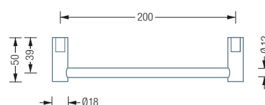
BG12-900E Draufsicht:
