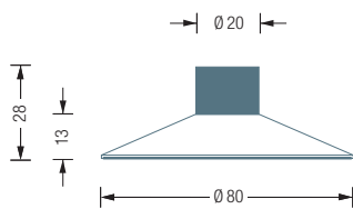
TSB80-13 Seitenansicht:
