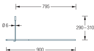
DSB300-900 Seitenansicht:
