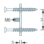
R55S Seitenansicht:
