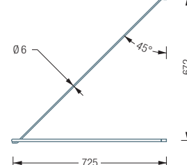
DR700HW Seitenansicht:
