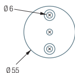
R55S Draufsicht:
