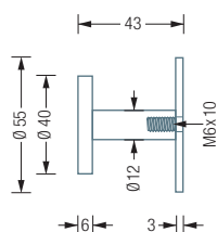
HA3-R55S55 Seitenansicht:
