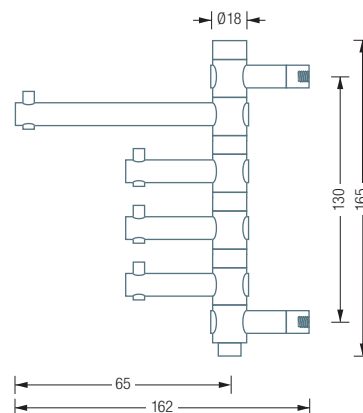
GH4-2 Seitenansicht:
