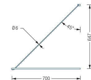
DSU1700-700W Seitenansicht:
