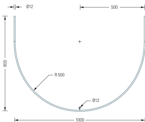
DR500HD800 Draufsicht:
