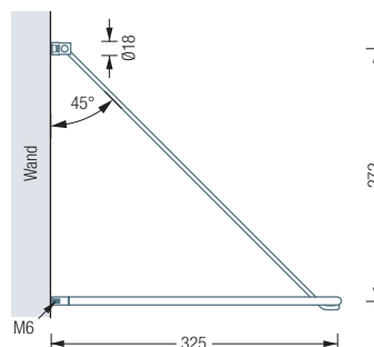
G300HW Seitenansicht:
