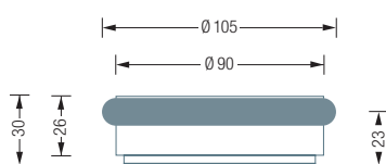
TSB90-30 Seitenansicht:
