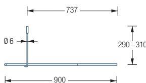
DSB500-900 Seitenansicht:
