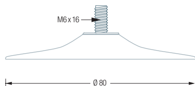
SN80-16/SN80-16S Seitenansicht:
