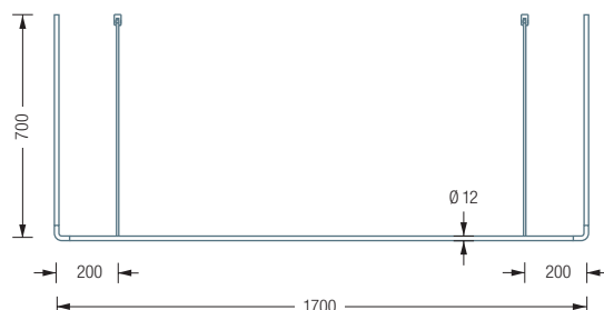
DSU1700-700W Draufsicht:
