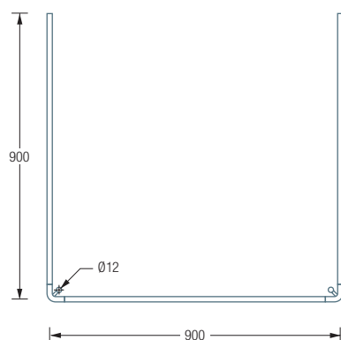
DSU900-900 Seitenansicht:
