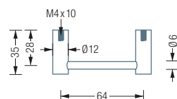
BG6-288E Draufsicht:
