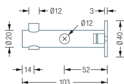
G9-600 / 1200 Seitenansicht:
