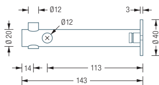
G4-600/1200 Seitenansicht:
