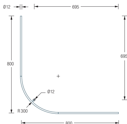
DSB300-800 Draufsicht:
