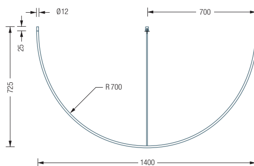
DR700HW Seitenansicht:
