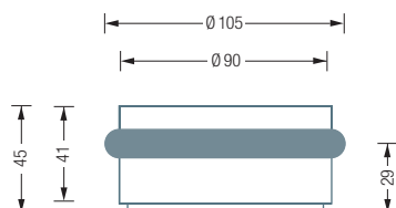
TSB90-45 Seitenansicht:
