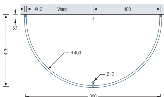
G400HD Draufsicht:
