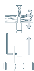
HG18-50D Schrankbodenmontage:
