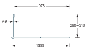
DR500HD1000 Seitenansicht:
