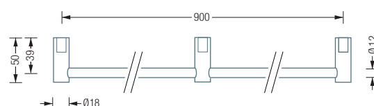
BG12-900E Draufsicht:
