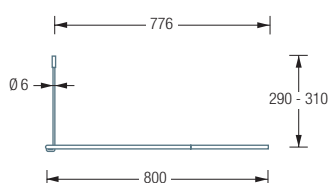
DR500HD800 Seitenansicht:
