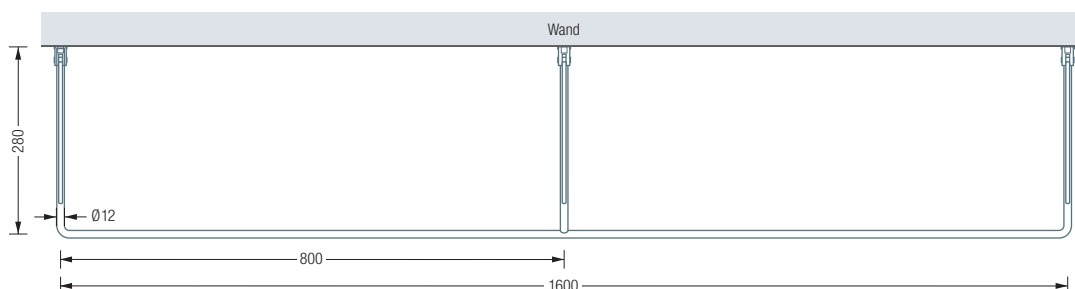
GU1-1600 Draufsicht:
