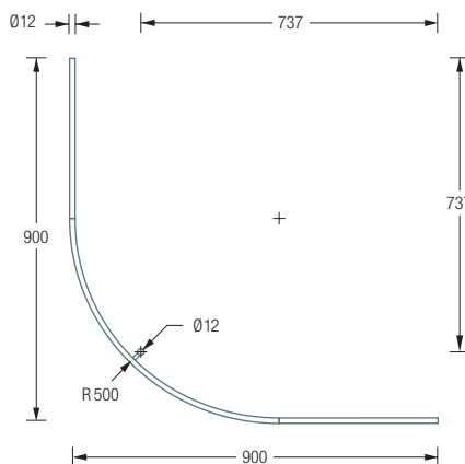
DSB500-900 Draufsicht:
