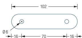
ROV23-B6 Draufsicht:
