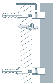
Fahnenmontage:
