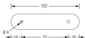
ROV23-B4 Draufsicht:
