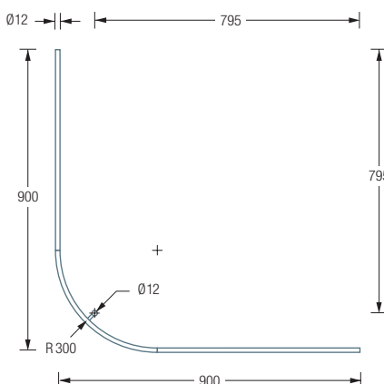
DSB300-900 Draufsicht:
