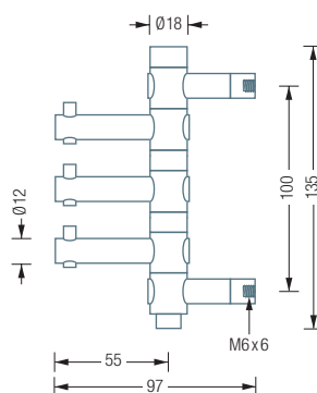
GH3 Seitenansicht:
