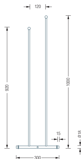
HTB2 Seitenansicht:
