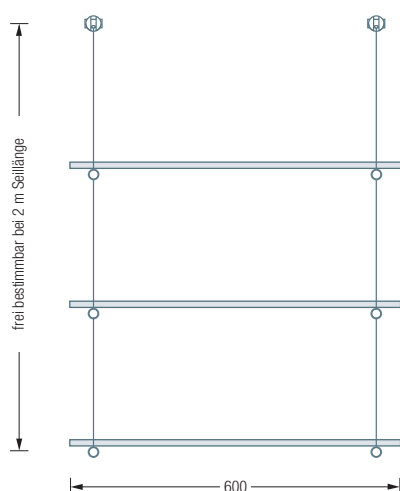
RST260-3 Frontansicht:
