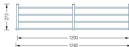
G8-1200 Draufsicht:
