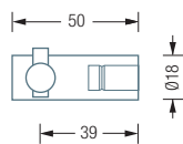
H18-50D Seitenansicht:
