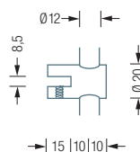
Detail Glasbodenträger:
