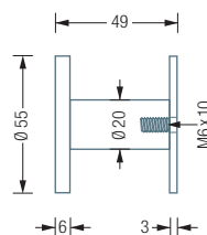
HA3-R55S55 Seitenansicht:
