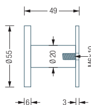
HA3-R55S55 Seitenansicht:
