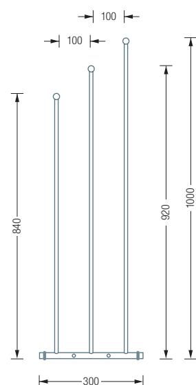
HTB3 Seitenansicht:
