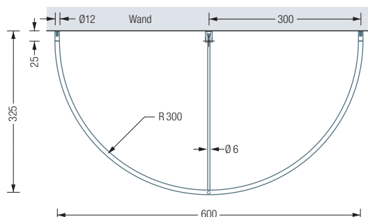
G300HW Draufsicht:
