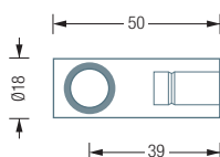
HG18-50D Seitenansicht:
