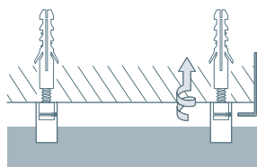
Deckenmontage:
